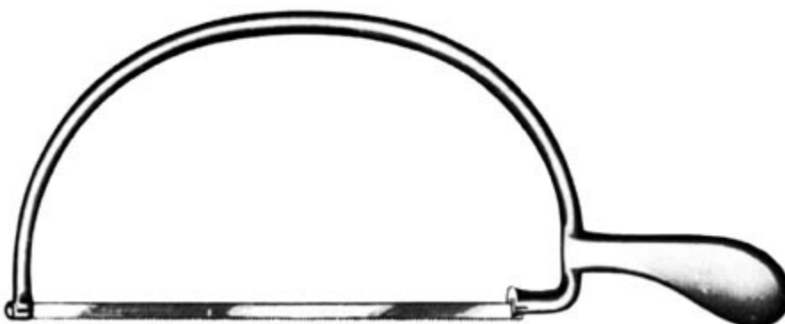
BIER 39-0440 35 cm, 14" mit je 1 Sägeblatt 4 mm, 6 mm und 8 mm with 1 each saw blade 4 mm, 6 mm and 8 mm con 1 hoja de 4 mm, 6 mm y 8 mm de cada una avec 1 lame de 4 mm, 6 mm et 8 mm de largeur
